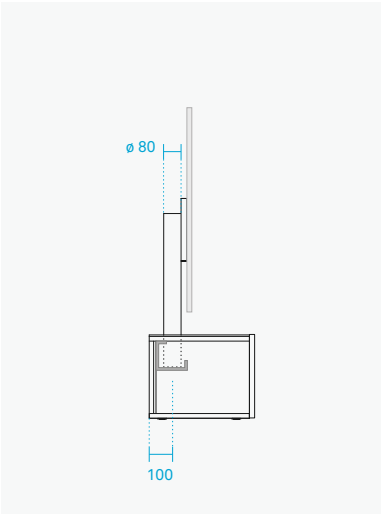
Supporto per TV sospesa possibile con ribalta o anta battente. Mounted TV stand possible with flap door or swing door.
