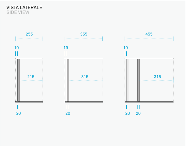
Spazio tecnico e schiena. Technical space and back panel.
