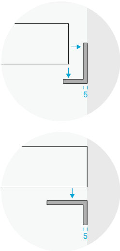
Profilo di sostegno Titanio Brunito. Due modalità di fissaggio a parete. Support profile Titanio Brunito. Two wall-mounting options.
