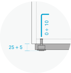
TAPPI COPRIFORO In colore uniforme alla struttura su Bianconeve, Rugiada, Fumo. In Titanio Brunito su Rovere, Noce, Eucalipto e Laccato Opaco Colore. HOLE COVER CAPS In a matching colour with the unit in Bianconeve, Rugiada, Fumo. In Titanio Brunito with Oak, Walnut, Eucalyptus and Matt Lacquered Color.
