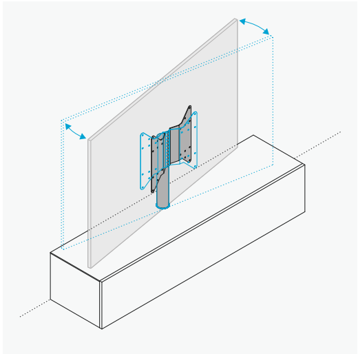
Per TV 55" e 65". Peso max 50 kg. For TV 55" e 65". Max. weight 50 kg.
