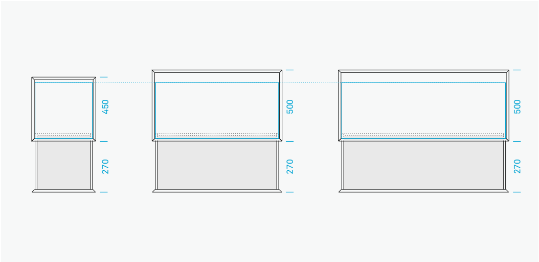
Estrazione totale. Interno Piqué. Fondo in Easy Pelle a richiesta. Total extraction drawers. Interior in Piqué. Bottom in Easy Leather on request.
